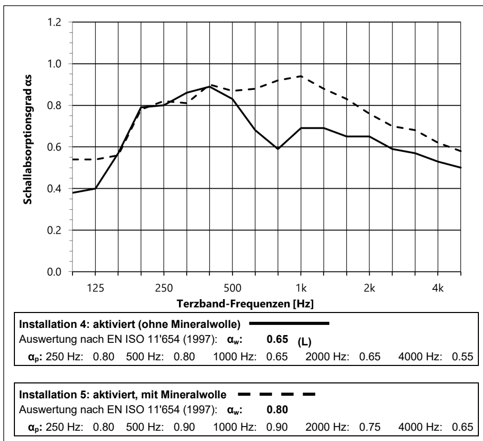
Abb. 9: Geschlossene Metall-Heiz-/Kühldecke mit Vlies (Installation 4) und mit zusätzlicher Mineralwolle (Installation 5)
