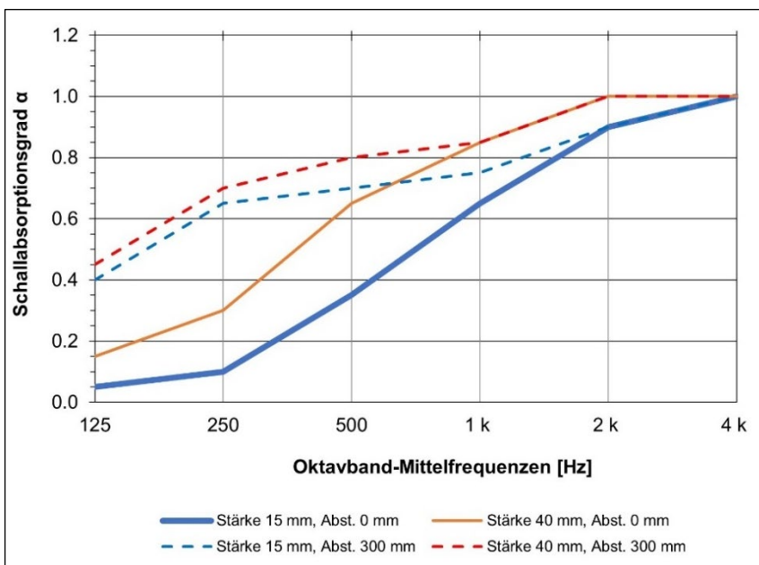
Abb. 6: Werte aus Fasold/Veres, Tabelle 4.3
