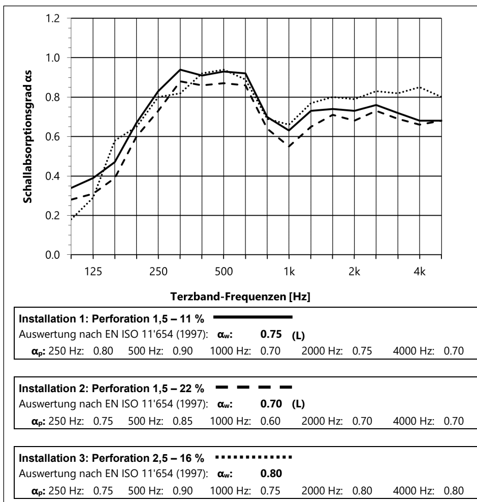
Abb. 8: Geschlossene Metalldecke mit Vlies und mit unterschiedlichen Perforationen (Angaben aus Produktunterlagen von Fural)
