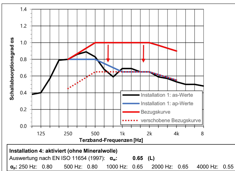
Abb. 12: Installation 4 von Abbildung 9 mit Bezugskurve zur Ermittlung des \alpha_w -Wertes
