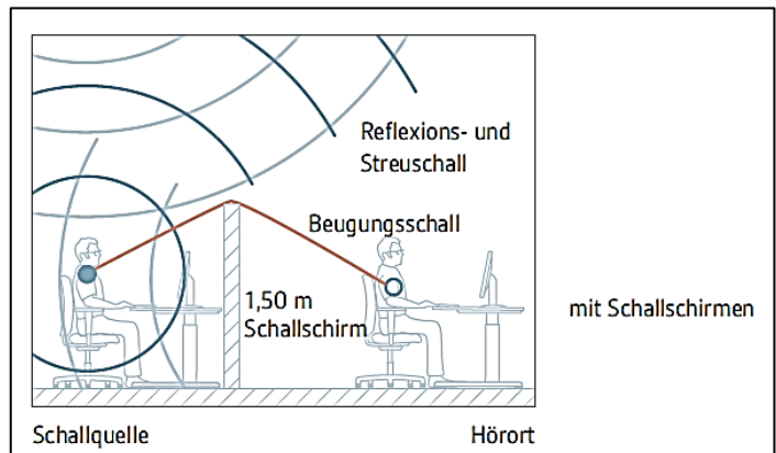
Abb. 2: Schallausbreitung im Mehrpersonenbüro mit Schallschirm (IBA)
