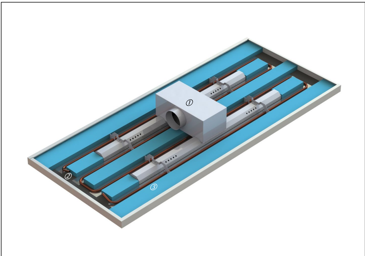
Abb. 5: Klimadeckensystem mit Zuluftelement ①, aufgeklebtem Vlies ② auf der Deckenplatte und Mineralwoll-Streifen in schwarzer PE-Folie ③ (zur besseren Erkennbarkeit in der Abbildung blau statt schwarz)
