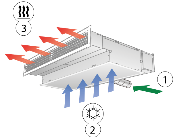
Figure 6. La fonction chauffage du PARAGON (à induction par eau) inclut également une fonction refroidissement
