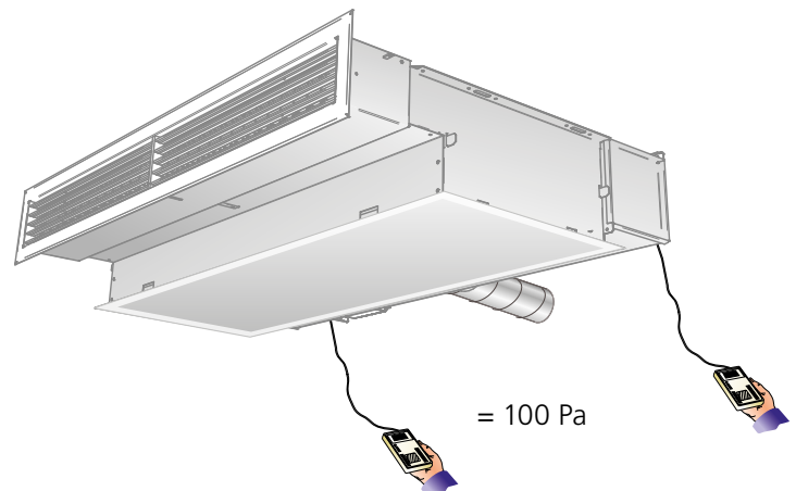
Figure 19. Emplacement des tubes de mesure
