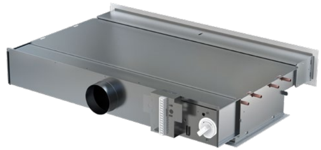
Figure 12. PARAGON avec raccordement hydraulique sur le côté droit.
