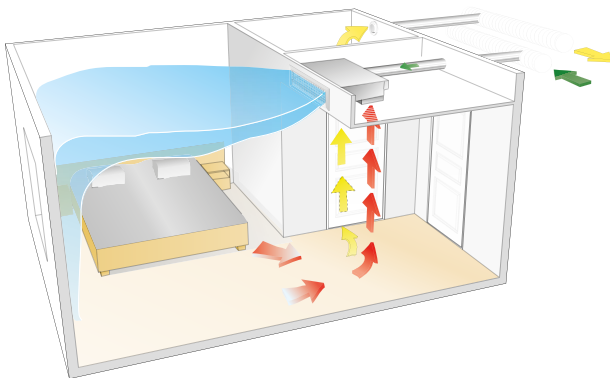
Figure 3 – Diffusion de l'air d'un module PARAGON dans une chambre d'hôtel
