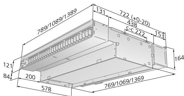
Figure 27. Schéma de dimensionnement sans grille
