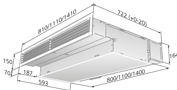
Figure 28. Schéma de dimensionnement avec grille
