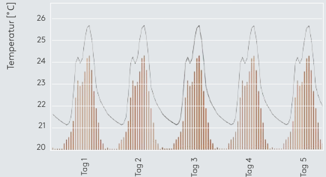
Temperaturverlauf im Raum bei Vollastbetrieb (Abb. 2)
