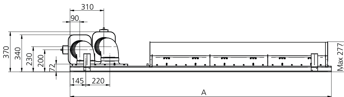
Figura 69. PACIFIC AM/AR con kit CAV, vista laterale con modulo di potenza nella versione destra.
