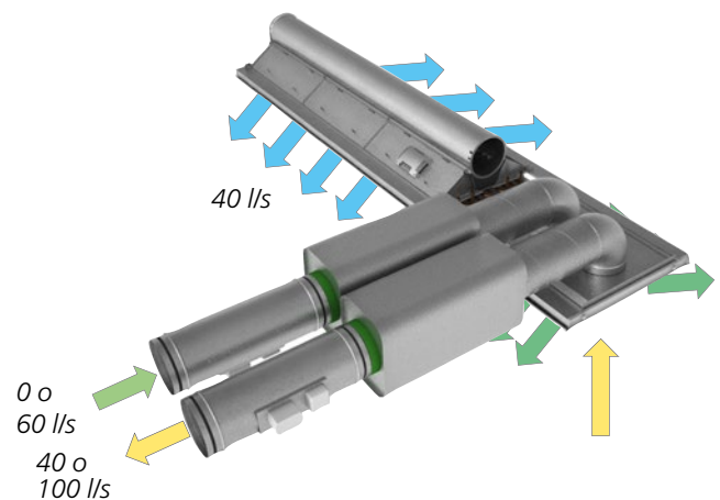
Figura 19. PACIFIC, con aria di mandata extra e aria di ripresa tramite T-AIR KIT VAV
