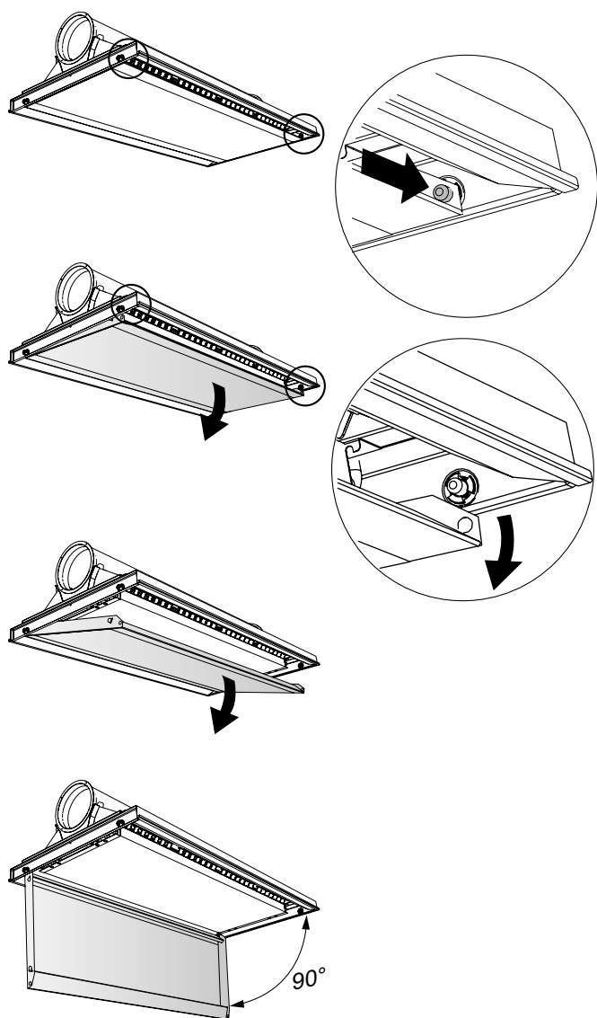
Figura 55. Apertura semplice della griglia di ricircolo mediante i cardini sul lato lungo opzionale.
