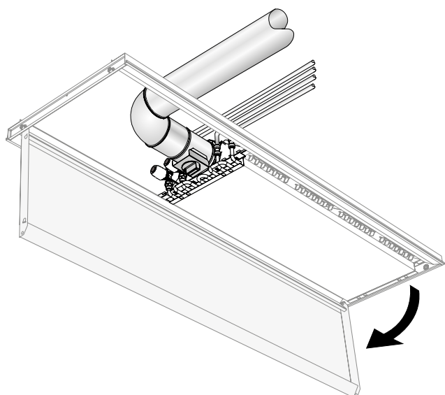
Figura 56. Esempio di accesso a una sezione inattiva con collegamenti orizzontali laterali quando la griglia di ricircolo viene aperta mediante i cardini.
