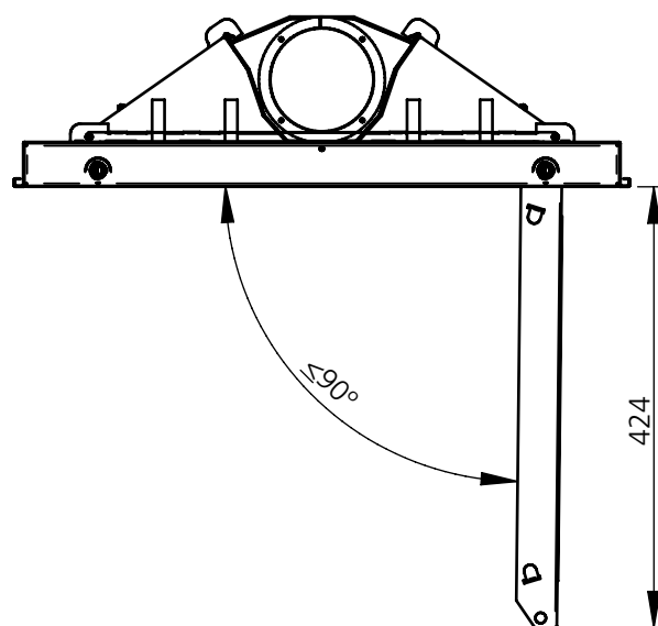
Figura 64. Schema delle quote della piastra anteriore con cerniere
