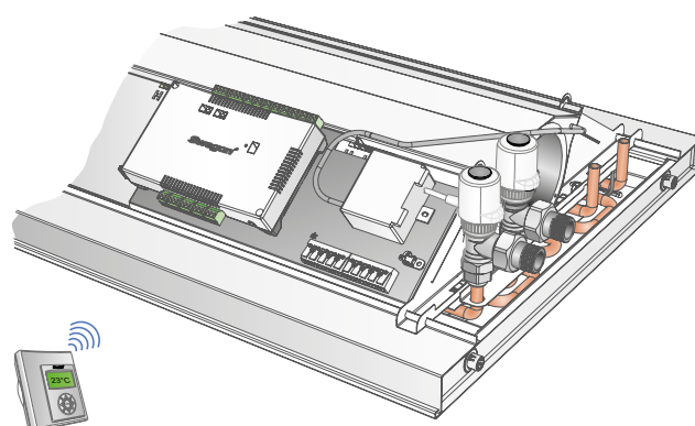
Figura 45. PACIFIC con regolatore Conductor installato e unità ambiente RU
