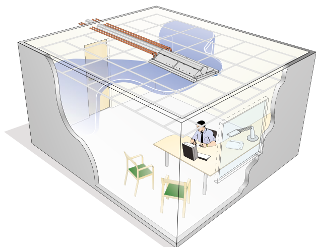
Figura 29. VariFlow con distribuzione dislocata della portata d'aria
