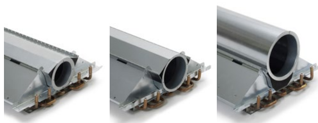
Figura 9. Modulo di potenza - Ø100; Ø125 e Ø160 mm
