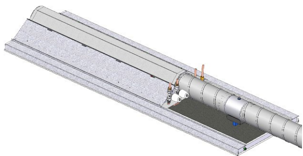
Figura 49. Esempio di raccordo dell'aria diritto e raccordi dell'acqua verticali.
