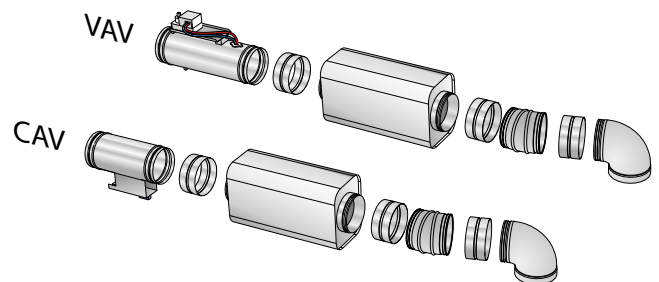
Figura 48. Installazione del kit AM/AR, VAV con controllo del motore e CAV con pomello manuale.
