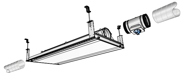
Figura 46. Variante di sospensione rispettivamente con staffe di montaggio e aste filettate.
