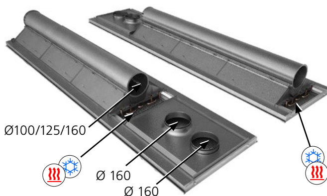
Figura 10. PACIFIC AM/AR con modulo di potenza e AM/AR aggiuntivo - Ø160 mm, due opzioni per i punti di allacciamento per i tubi di raffreddamento e riscaldamento.
