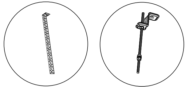
Figura 46. Variante di sospensione rispettivamente con staffe di montaggio e aste filettate.
