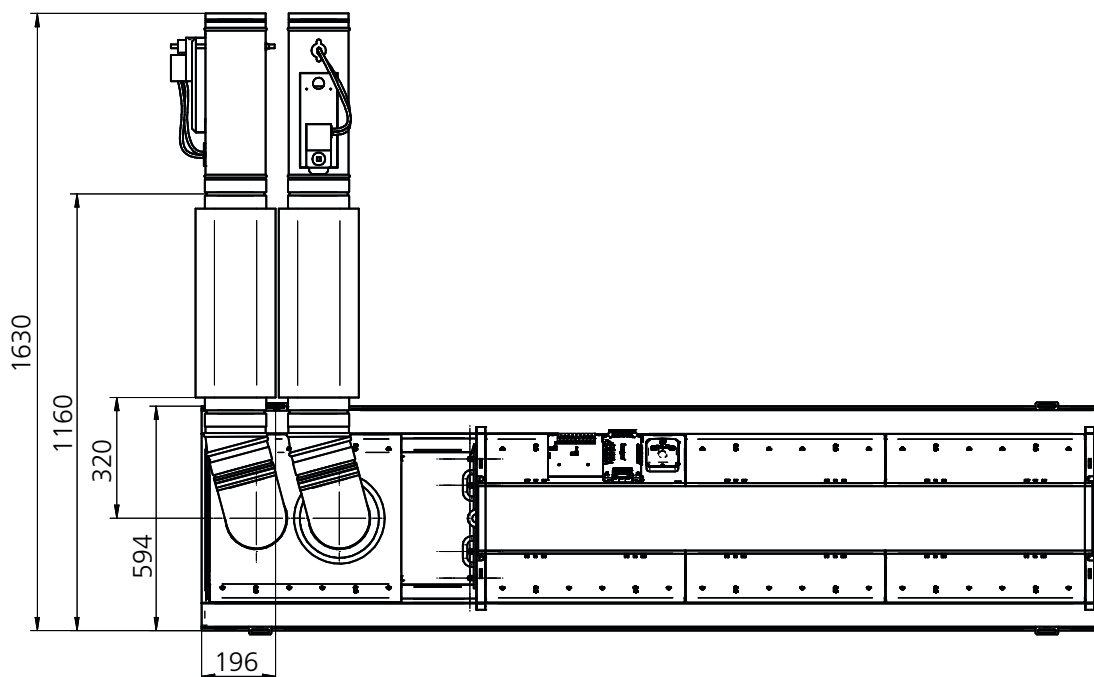
Figura 68. PACIFIC AM/AR con kit VAV, vista dall'alto con modulo di potenza nella versione destra.
