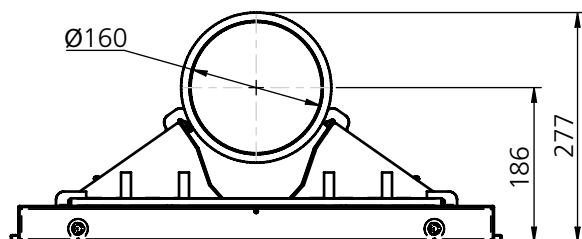
Figura 61. Schema delle quote – raccordo dell'aria
