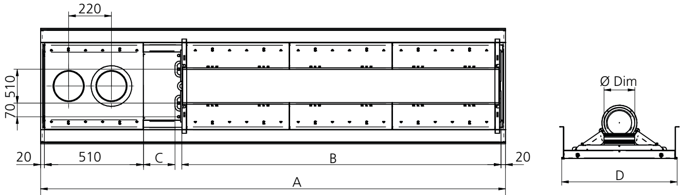
Figura 66. PACIFIC AMIAR, vista dall'alto con modulo di potenza nella versione destra e vista con la parete terminale.
