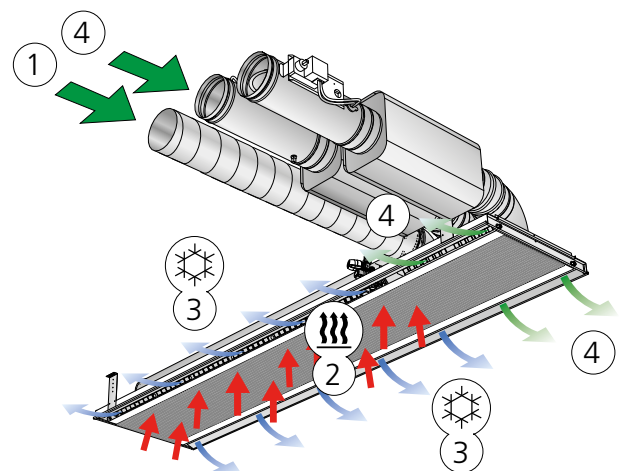
Figura 7. Funzione di raffreddamento per PACIFIC AMIAR
