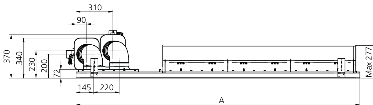
Figura 67. PACIFIC AM/AR con kit VAV, vista laterale con modulo di potenza nella versione destra.
