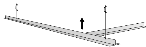
Figura 47. Installazione dell'unità PACIFIC con sospensione mediante aste filettate.
