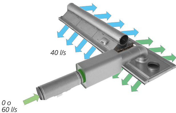
Figura 18. PACIFIC, con aria di mandata extra tramite AIR KIT VAV
