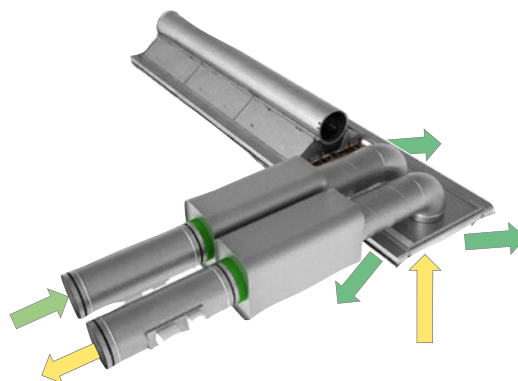
Figura 17. PACIFIC, con aria di mandata extra e aria di ripresa tramite T-AIR KIT CAV
