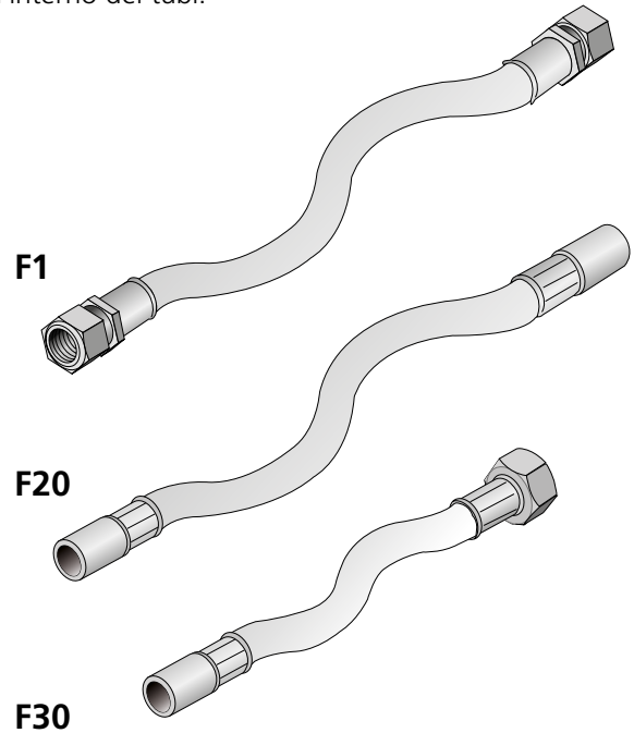
Figura 41. Tubi di collegamento flessibili, SYST FH
