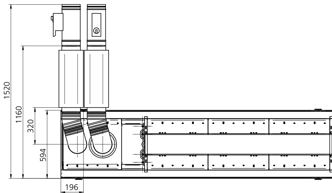
Figura 70. PACIFIC AM/AR con kit CAV, vista dall'alto con modulo di potenza nella versione destra.
