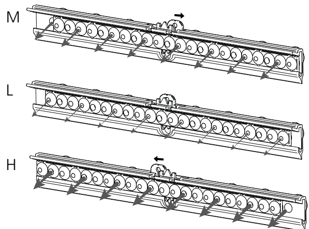
Figura 26. Striscia di ugelli VariFlow impostata in tre posizioni. L, M e H
