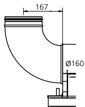
Figura 63. Schema delle quote – raccordo dell'aria verticale con gomito
