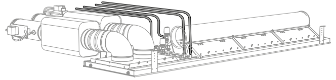
Figura 13. Pacific AM/AR con tubi per l'acqua collegati tra il modulo di potenza e il modulo AM/AR.
