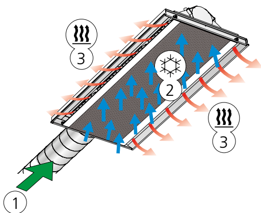
Figura 5. Funzione di riscaldamento
