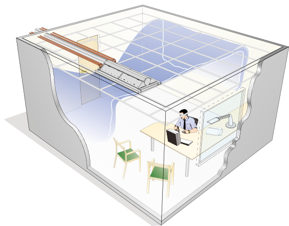
Figura 27. VariFlow con distribuzione asimmetrica della portata d'aria
