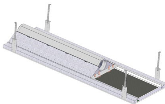
Figura 53. Esempio di sospensione della trave con fascette di montaggio.
