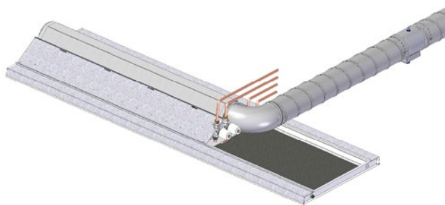
Figura 50. Esempio di raccordi dell'aria e dell'acqua laterali.
