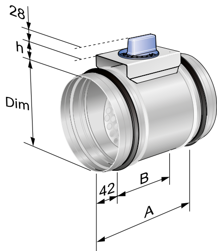
Figura 35. Serranda di taratura SYST CRPc 9-100, 125 o 160
