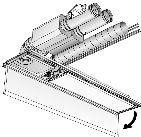
Figura 58. Esempio di accesso a un'unità PACIFIC AMIAR con kit VAV quando la griglia di ricircolo viene aperta mediante i cardini.
