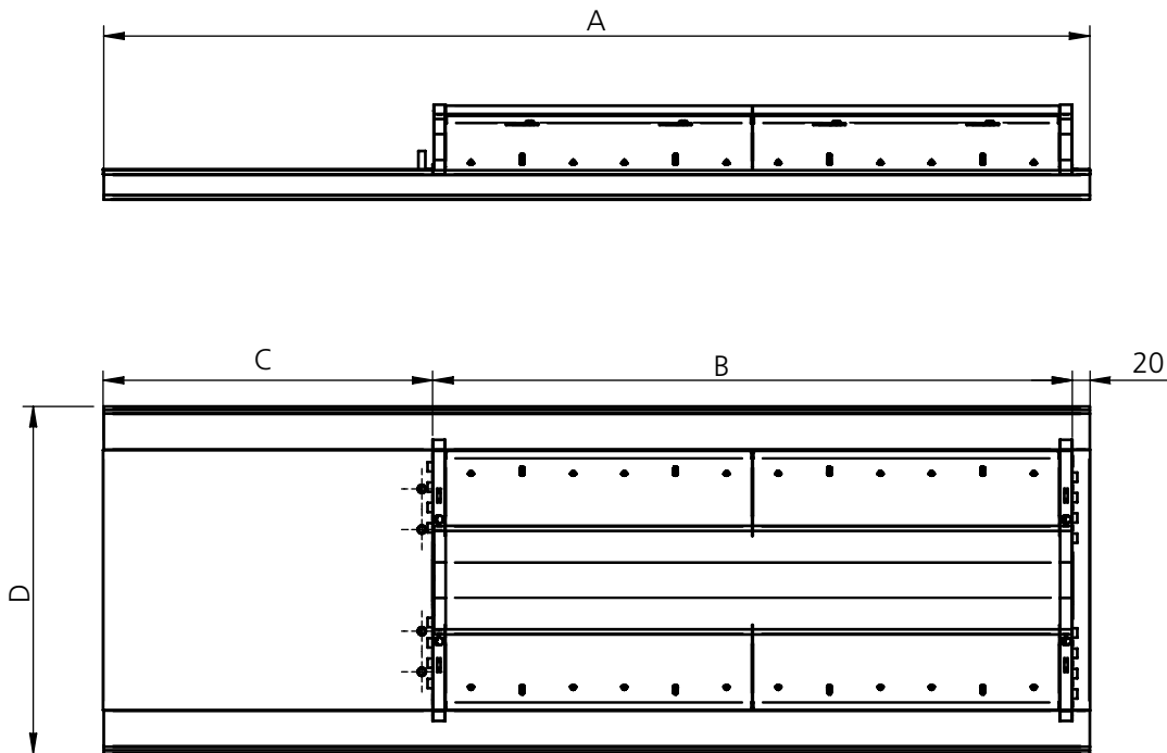
Figura 60. Schema delle quote relativo al modulo di design con profili a T con distanza di 600 mm da centro a centro, con modulo di potenza nella versione destra – Vista laterale e dall’alto
