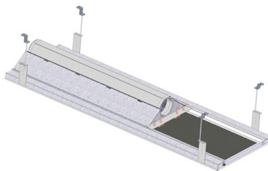
Figura 52. Esempio di sospensione della trave con aste filettate.
