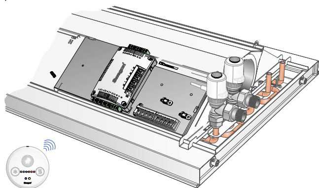
Figura 43. PACIFIC con regolatore URC1 e modulo del sensore installato.
