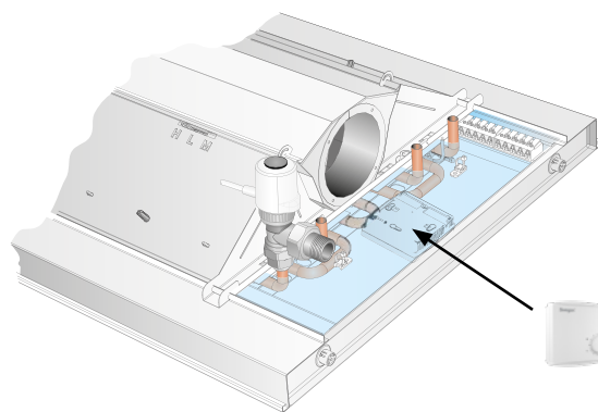
Figura 44. PACIFIC con regolatore LUNA installato.
