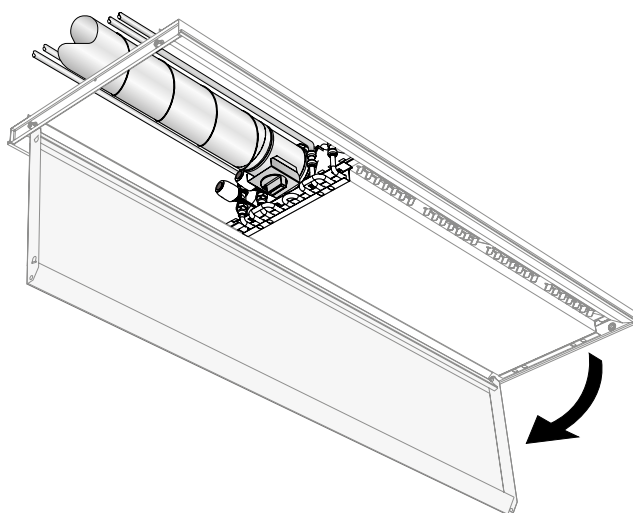
Figura 57. Esempio di accesso a una sezione inattiva con collegamenti orizzontali dritti quando la griglia di ricircolo viene aperta mediante i cardini.
