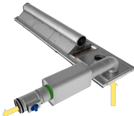
Figura 16. PACIFIC, con aria di ripresa tramite T-AIR KIT CAV
