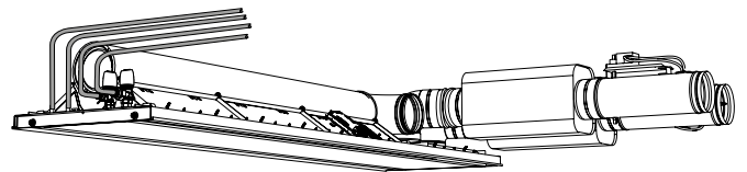
Figura 14. Pacific AM/AR con tubi per l'acqua collegati sul lato corto.
