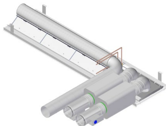
Figura 54. Esempio con PACIFIC AMIAR incl. kit CAV con raccordi dell'aria e dell'acqua laterali.
