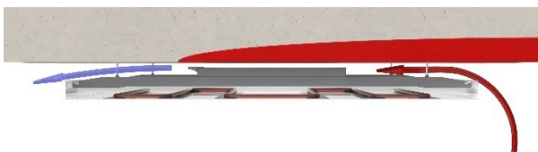
Fig. 5: Fonctionnement du canal de buses Barcol-Air
