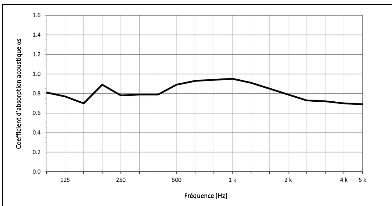
Fig. 6: Courbe d'absorption acoustique sur différentes fréquences, exemple d'un plafond climatisé en métal avec non-tissé acoustique et matelas en laine minérale
