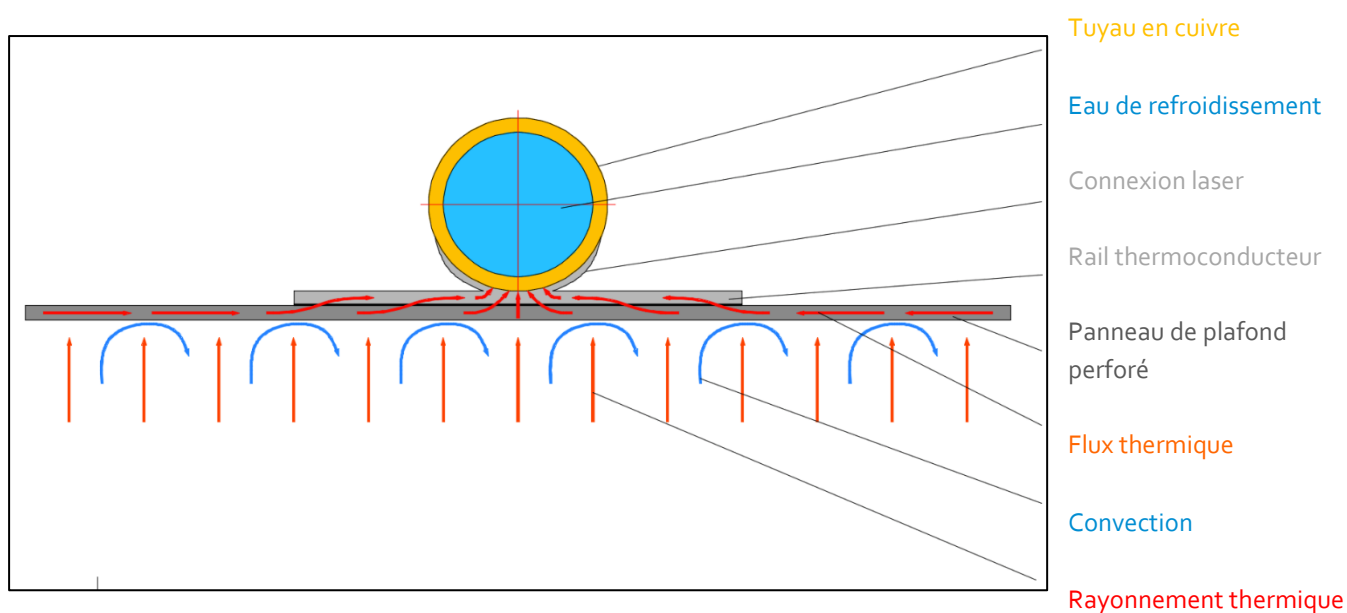
Fig. 1: Fonctionnement de base d'un plafond climatisé
