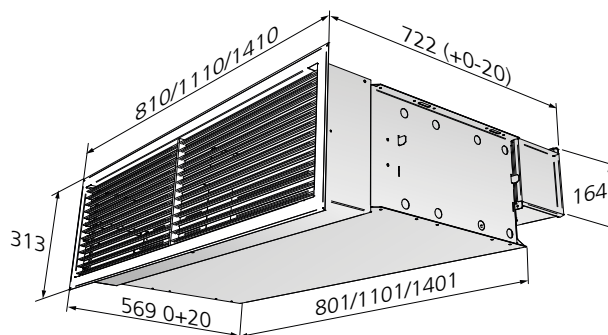
Figure 25. Schéma de dimensionnement avec grille
