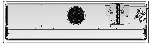
Figure 19. Raccordement hydraulique centré au dos.
