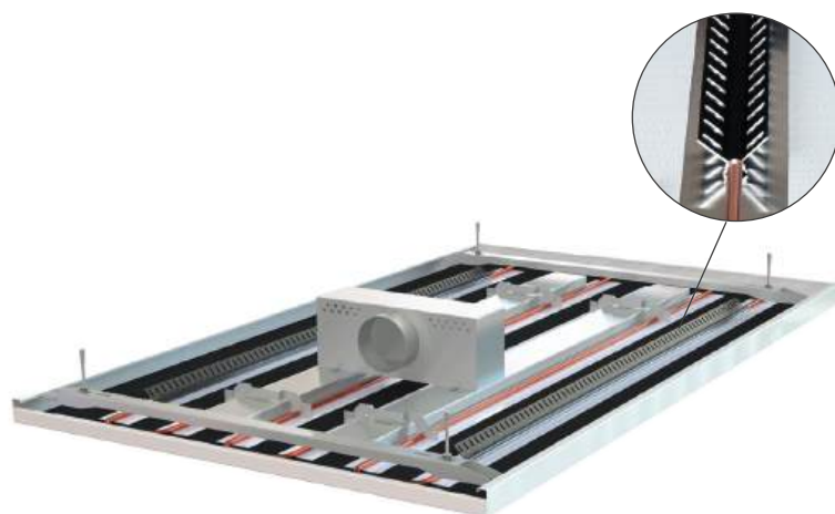
Les panneaux de plafond A11-S activés conviennent à l'utilisation de Convector Wings.
