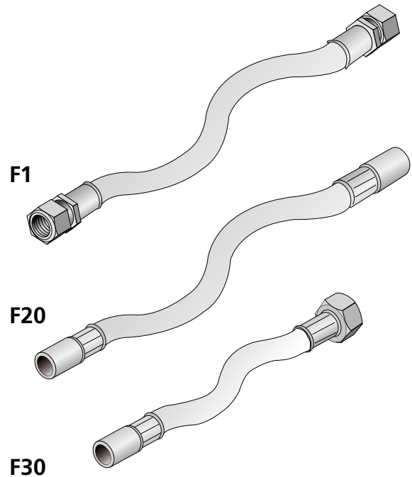
Abbildung 41. Flexible Anschlussschläuche, SYST FH
