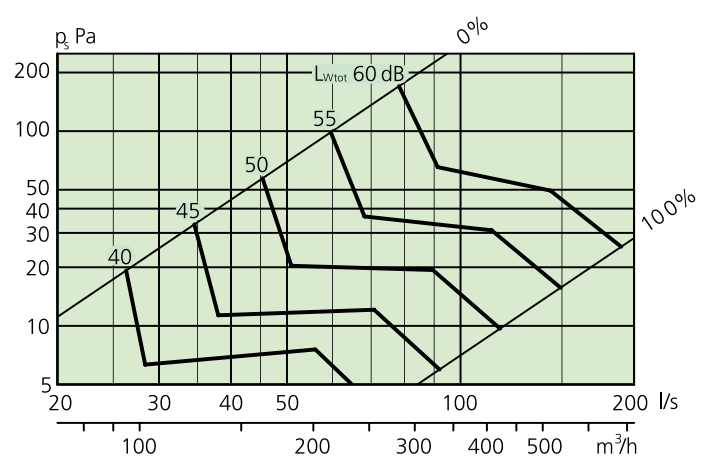
Diagramm 9. Einstückerbereich, Klappe SYST CRPc 9-160
