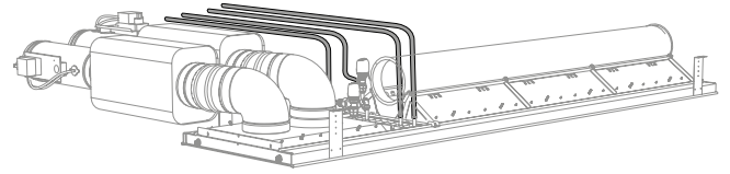
Abbildung 13. Pacific SA/EA mit Wasseranschluss zwischen Leistungsmodul und SA/EA-Modul.
