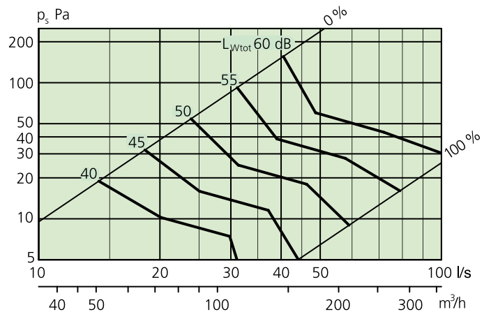
Diagramm 8. Einstückerbereich, Klappe SYST CRPc 9-125
