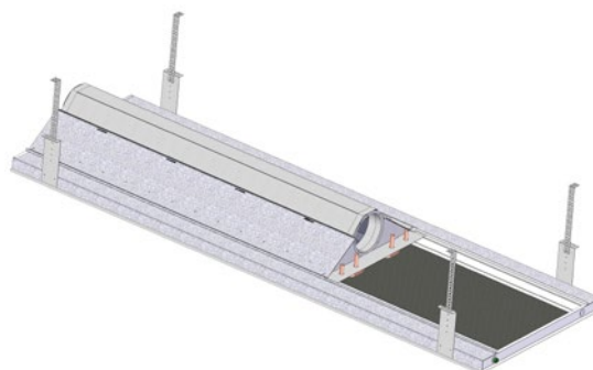
Abbildung 53. Beispiel einer Aufhängung mit Montageband.
