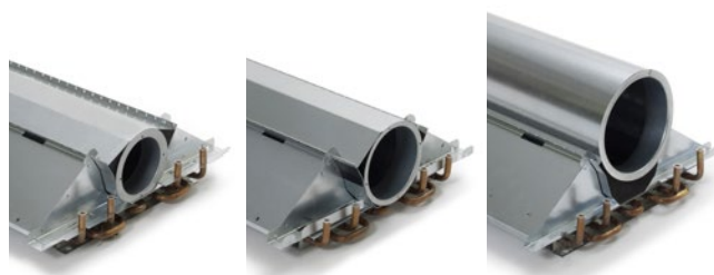
Abbildung 9. Leistungsmodul - Ø100, Ø125 und Ø160 mm
