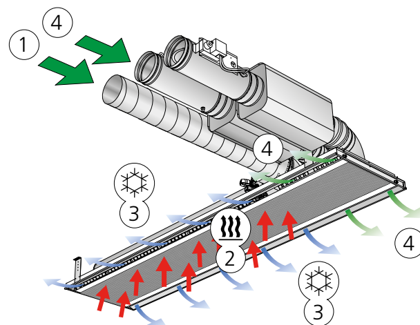
Abbildung 7. Kühlfunktion für Pacific SA/EA
