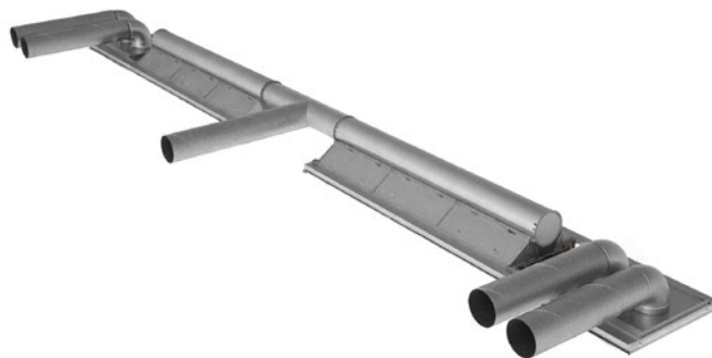
Abbildung 22. Paarweise Kupplung zweier PACIFIC SA/EA
