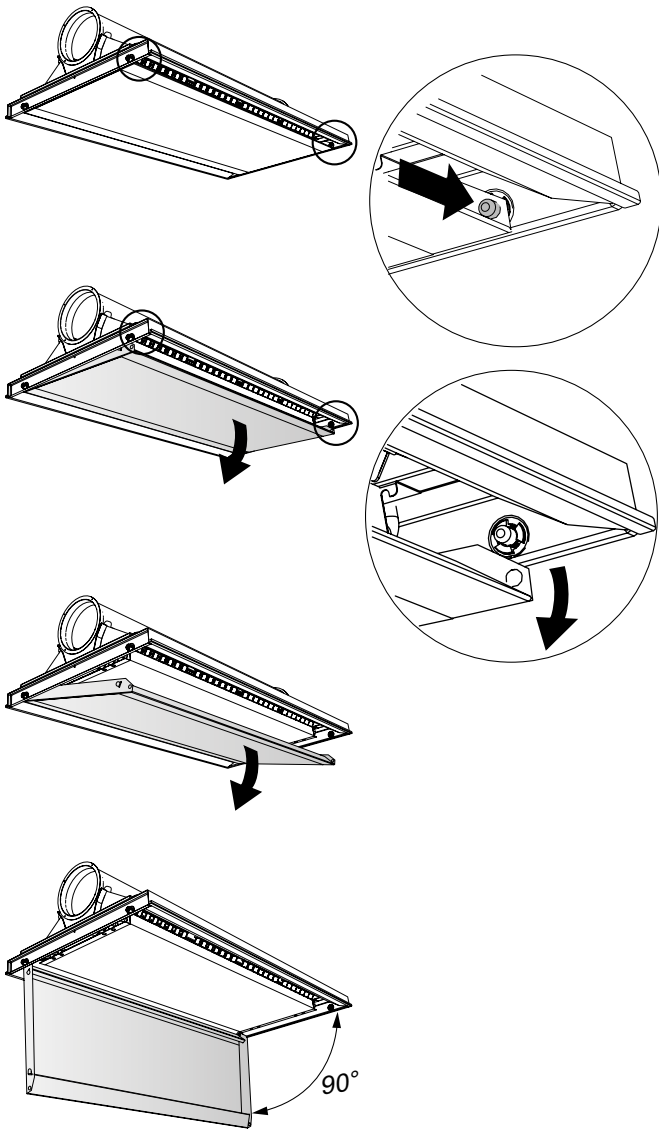
Abbildung 55. Einfaches Klappen des Unterblechs an wahlfreier Längsseite.
