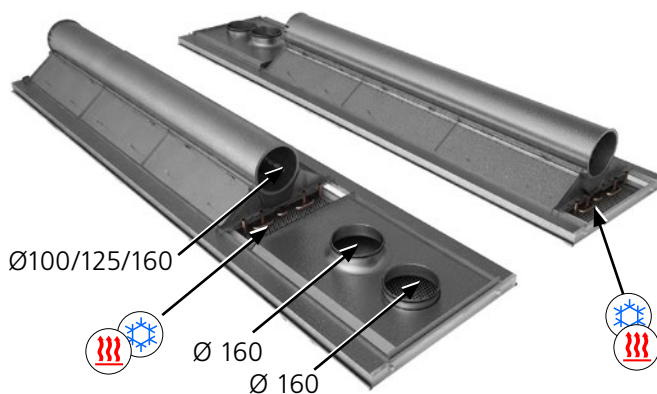
Abbildung 10. PACIFIC SA/EA mit Leistungsmodul und Zusatzmodul SA/EA - Ø160 mm, zwei Anschlusspunkialternativen für Kühl- und Heizrohr.
