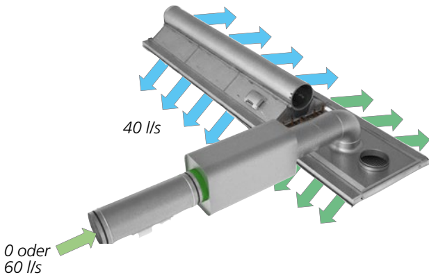
Abbildung 18. Pacific mit zusätzlicher Zuluft über Air Kit VAV
