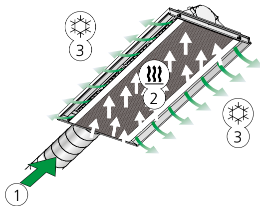
Abbildung 6. Neutralfunktion
