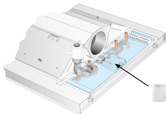
Abbildung 44. Pacific mit montierter Steuerausrüstung LUNA
