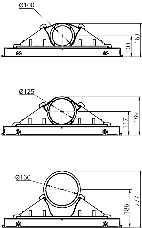
Abbildung 61. Maßskizze - Luftanschluss
