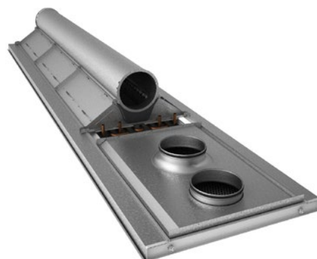
Abbildung 3. Pacific mit Zusatzmodul SA/EA.
