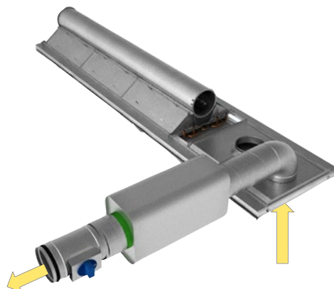
Abbildung 16. Pacific mit Abluft über T-AIR KIT CAV
