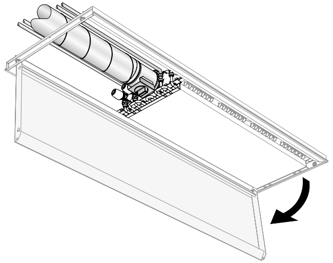
Abbildung 57. Beispiel für den Zugang bei inaktivem Teil und geradem horizontalem Anschluss bei heruntergeklapptem Unterblech.
