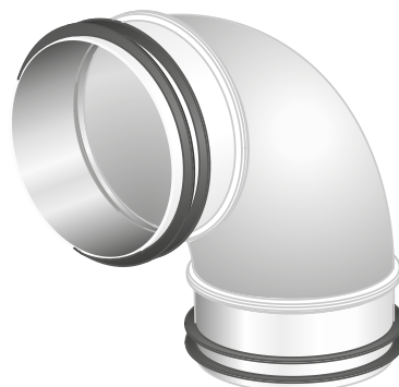
Abbildung 36: Anschlussdetail Luft - Kanalbogen 90°, SYST CA 100/125/160-90
