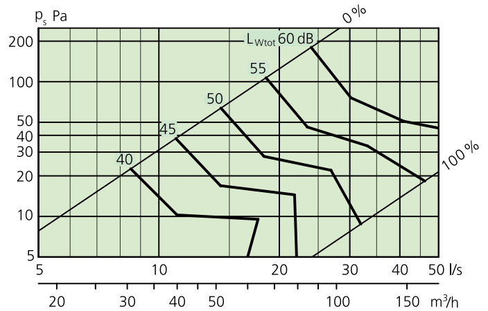
Diagramm 7. Einstückerbereich, Klappe SYST CRPc 9-100
