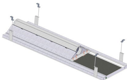
Abbildung 52. Beispiel einer Aufhängung mit Gewindestange.
