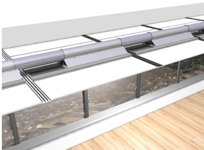
Abbildung 21. Mehrere in Serie gekuppelte PACIFIC (ohne Zusatzmodul SA/EA).
