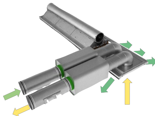
Abbildung 17. Pacific mit zusätzlicher Zuluft und Abluft über T-AIR KIT CAV
