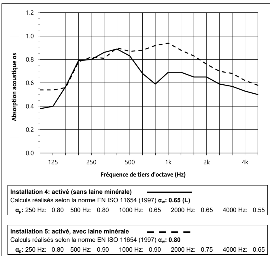
Fig. 9: Plafond métallique sous pression rafraîchissant/chauffant en non-tissé (Installation 4) et avec laine minérale supplémentaire (Installation 5)
