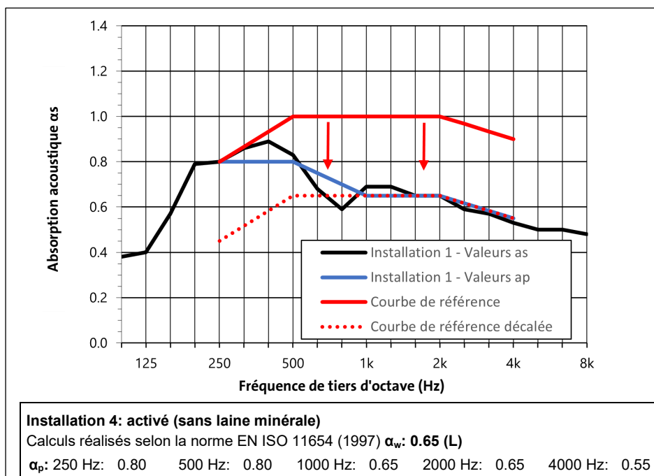
Fig. 12: Installation 4 de l'illustration 9 avec courbe de référence de la détermination de la valeur \alpha_w
