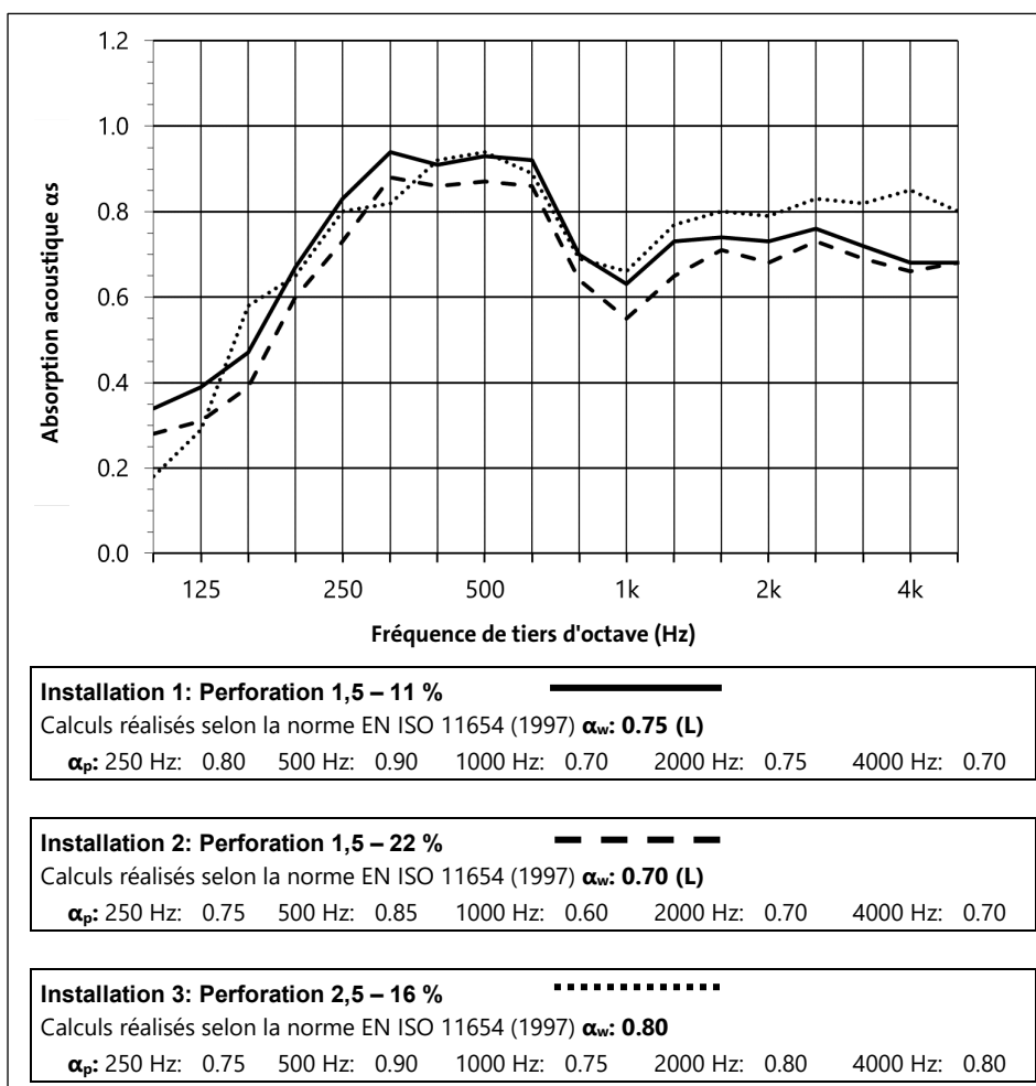
Fig. 8: Plafonds métalliques sous pression en non-tissé avec différentes perforations (chiffres issus de la documentation produit de Fural)
