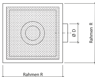
Typ D21-G Ausführung: quadratischer Rahmen
